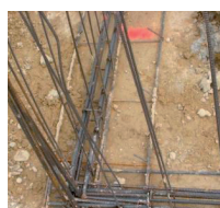
Nœud de chaînage - Continuité mécanique
