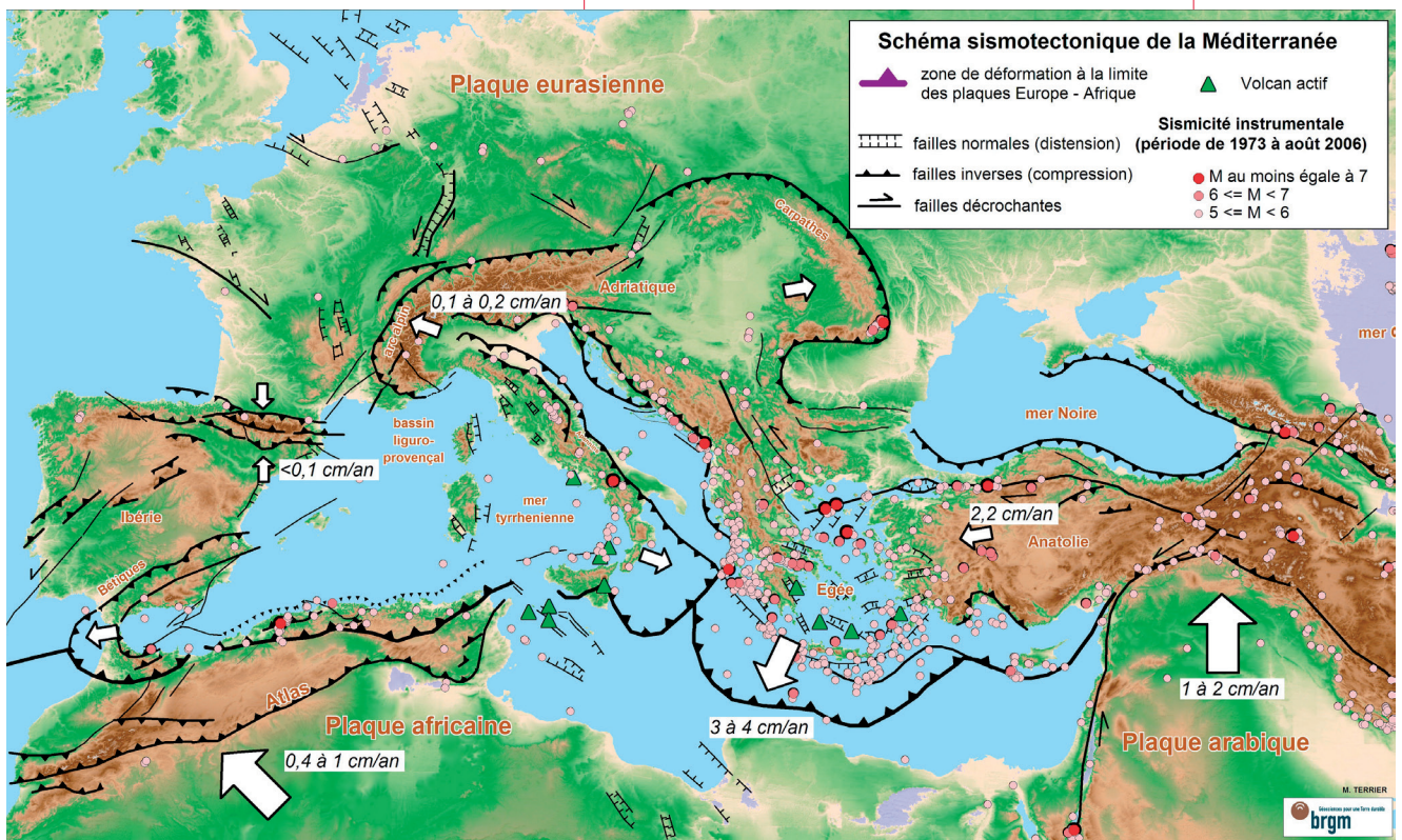
Schéma sismo-tectonique de la Méditerranée, M.Terrier (2006)
